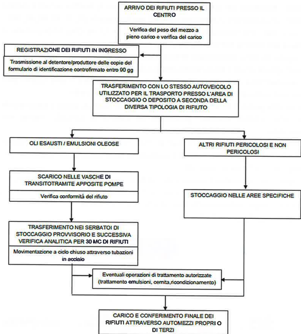
Figura 3 – Ciclo produttivo
